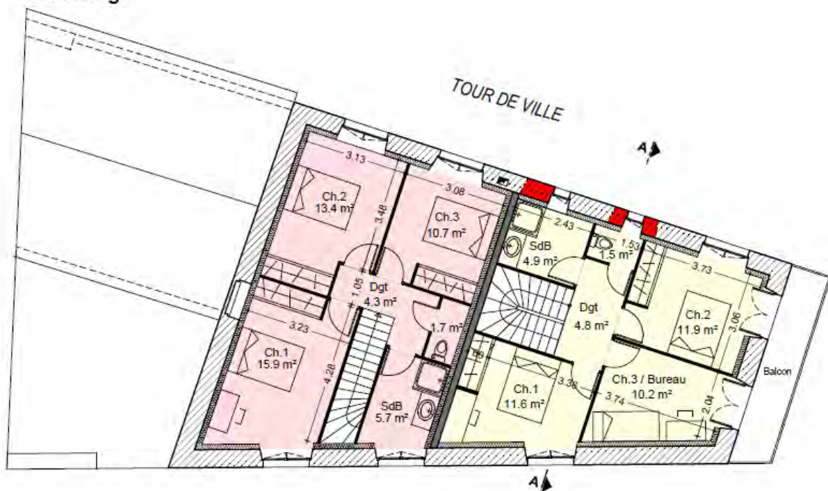
Plan Etage
